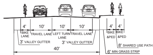
SECTION K - K'
